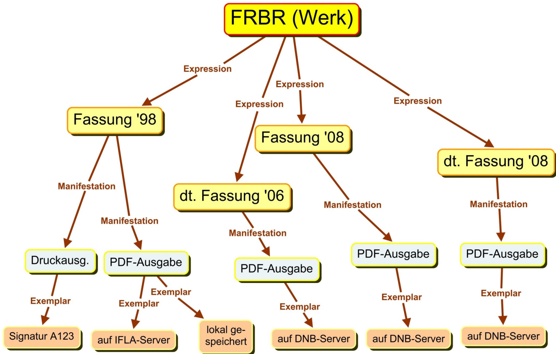
FRBR-Baum: am Beispiel des Werks „FRBR“ (Ausschnitt)
